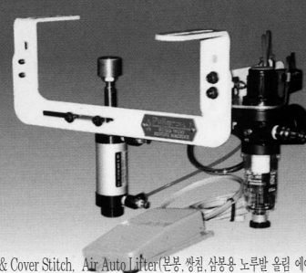
OPTION 1.2-Needle & Cover Stitch, Air Auto Lifter (본봉, 쌍침, 삼봉용 노루발 올림 에어장치)
