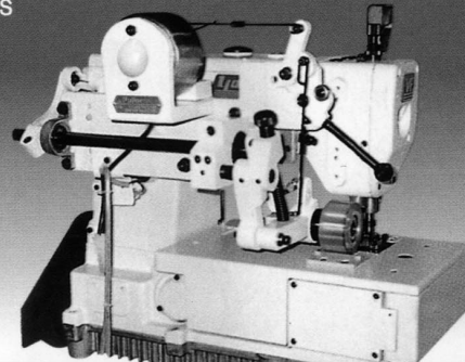
▲CV-S YAMATO 1500 Flat Bed, Solenoid Type, (평베드 삼봉, 솔자동)
