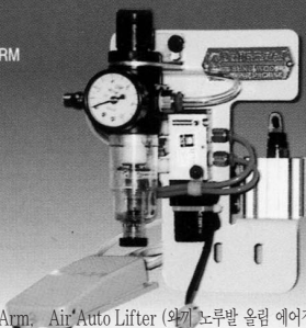
OPTION Feed-off-Arm, Air Auto Lifter (외개 노루발 올림 에어장치)
